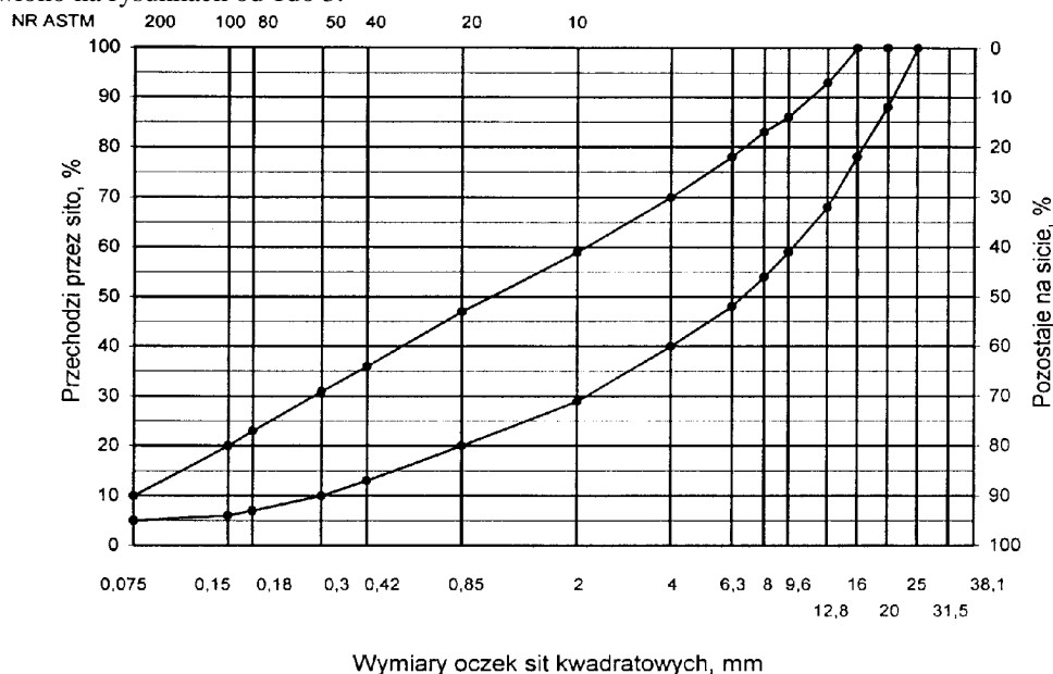
Rys. 1. Krzywe graniczne uziarnienia mieszanki mineralnej BA od 0 do 20 mm do warstwy ścieralnej nawierzchni drogi o obciążeniu ruchem dla KR1 lub KR280
