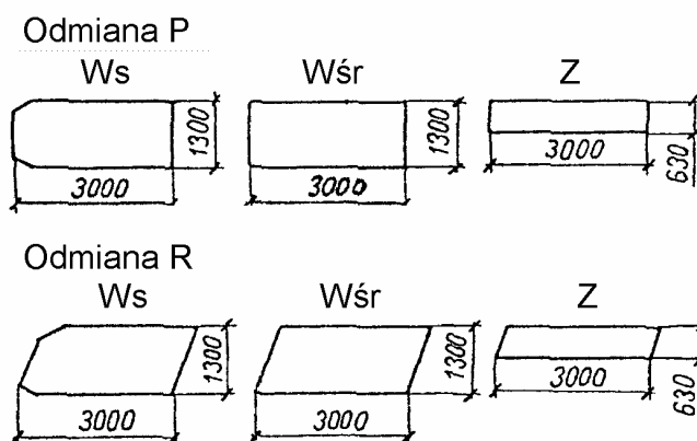
Rys. 1. Kształty, rodzaje i odmiany płyt
