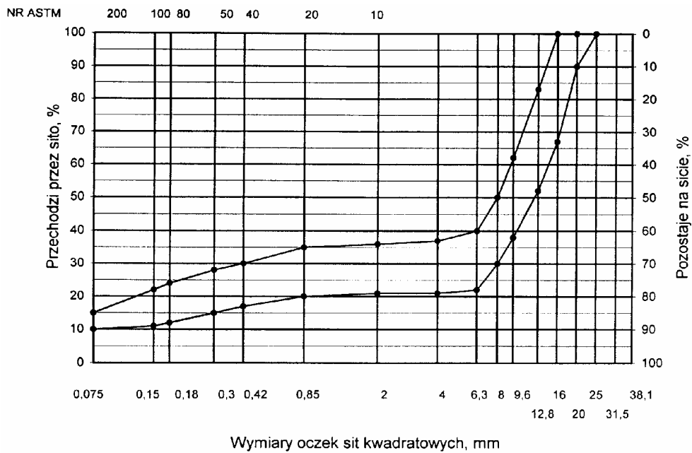
Krzywe graniczne uziarnienia mieszanki mineralnej BA od 0 do 20 mm (mieszanka o nieciąglym uziarnieniu) do warstwy ścieralnej nawierzchni
