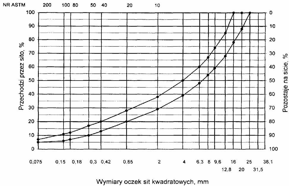
Krzywe graniczne uziarnienia mieszanki mineralnej BA od 0 do 20 mm do warstwy ścieralnej nawierzchni
