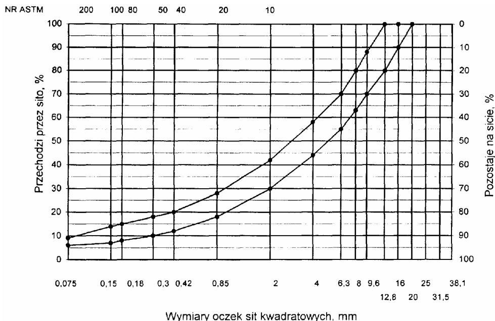
Krzywe graniczne uziarnienia mieszanki mineralnej BA od 0 do 16 mm do warstwy ścieralnej nawierzchni
